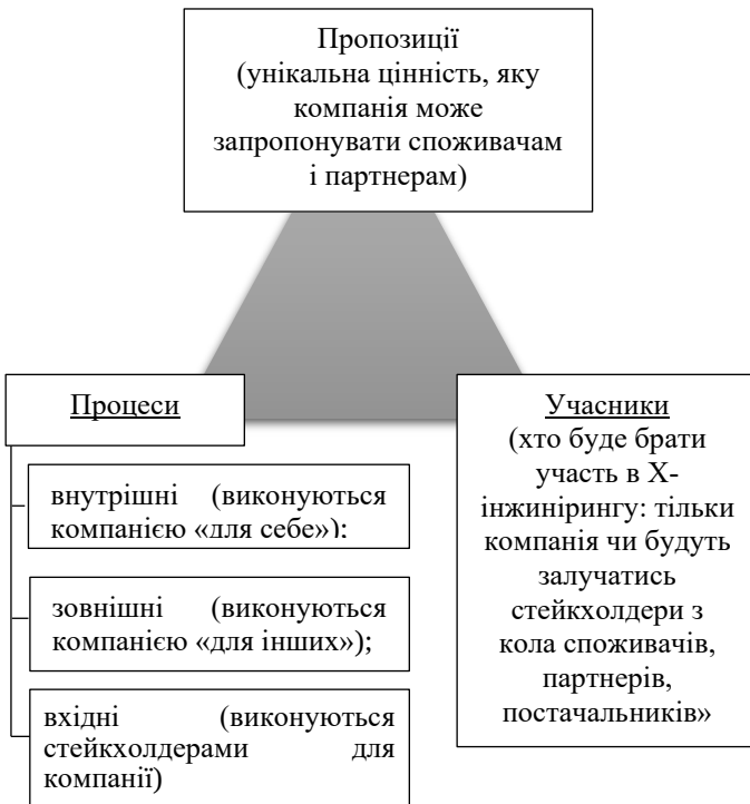
Рис. 5.18. Трикутник Х-інжинірингу
