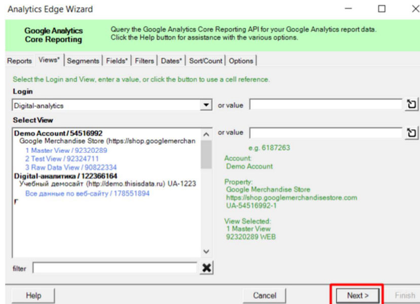
Рис. 5.42. Вкладка «Views»
