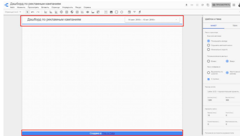
Рис. 6.28. Створення макету
