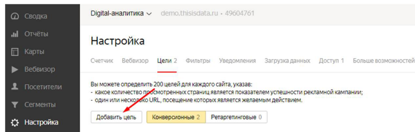
Рис. 4.45. Налаштування Метрики
