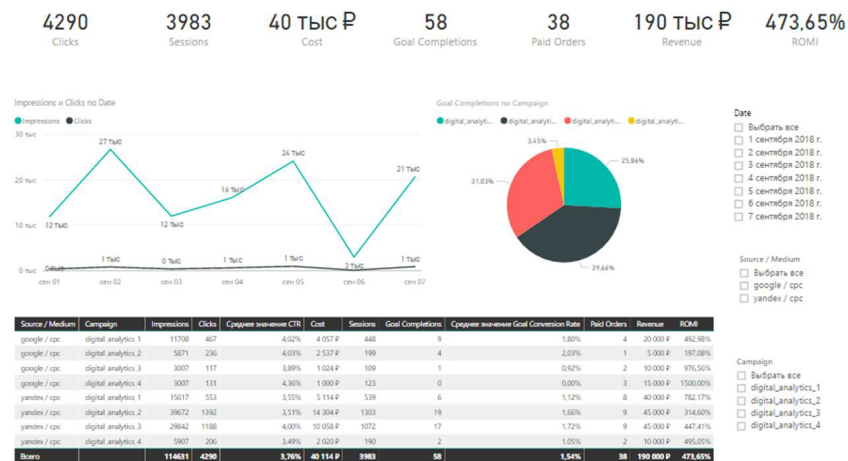
Рис. 6.51. Завершальний звіт
