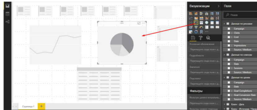
Рис. 6.42. Макет звіту
