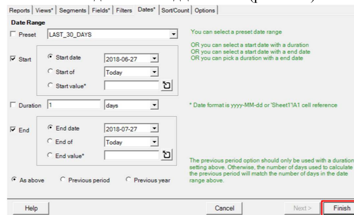
Рис. 5.44. Налаштування фільтра
