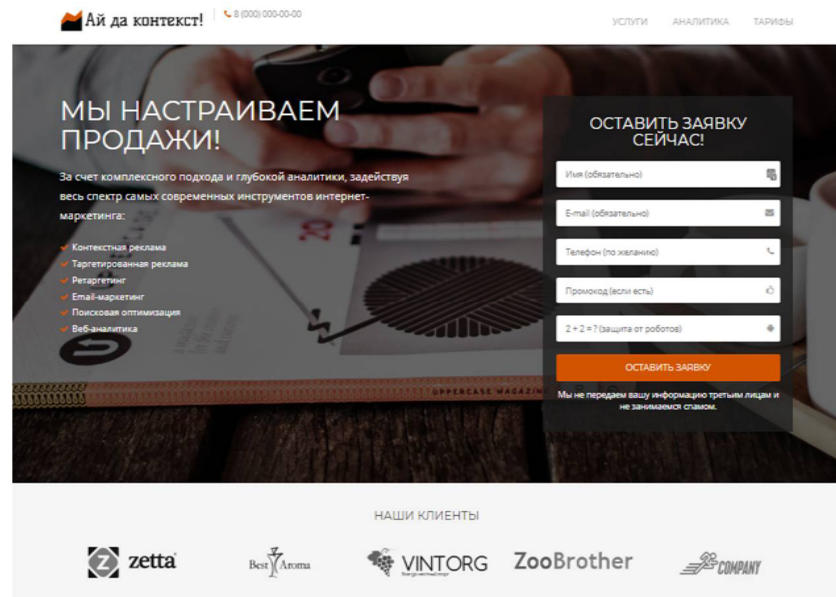
Рис. 3.24. Навчальний сайт
