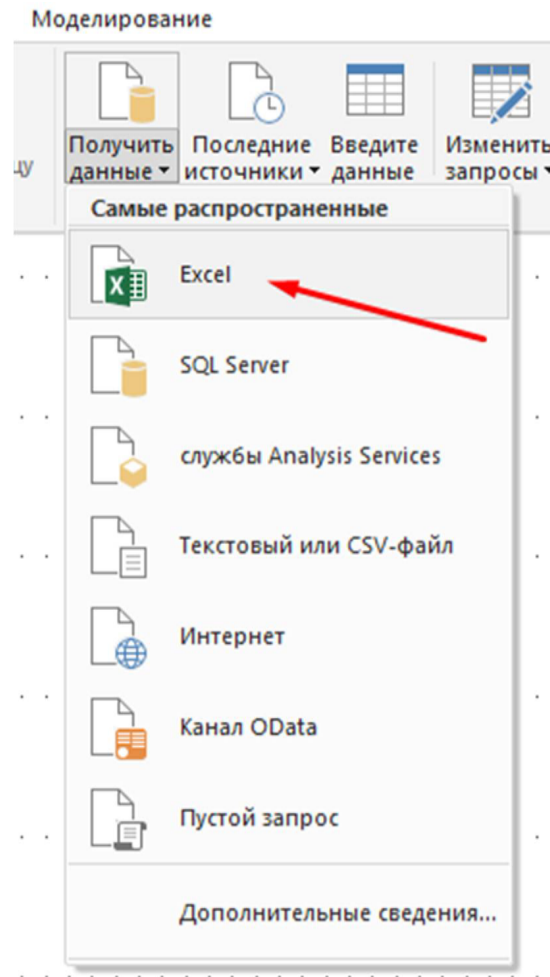
Рис. 6.42. Вибір конектора
