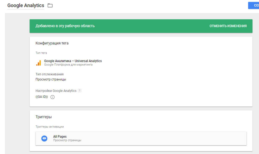
Рис. 4.18. Конфігурація тега
