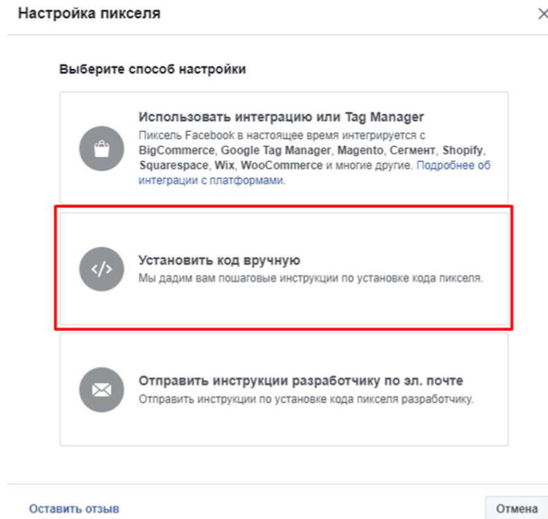
Рис. 4.23. Налаштування пікселя
